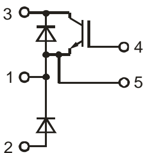
Рисунок 1 – Структурная схема модуля
