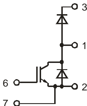
Рисунок 1 – Структурная схема модуля
