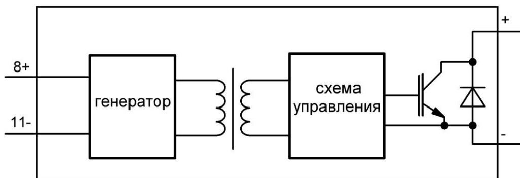
Рисунок 1 – Структурная схема модуля
