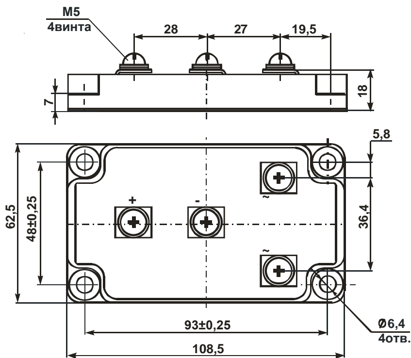
Неуказанные предельные отклонения присоединительных размеров \pm 0,5 мм Рисунок 2 – Габаритные и присоединительные размеры модуля
