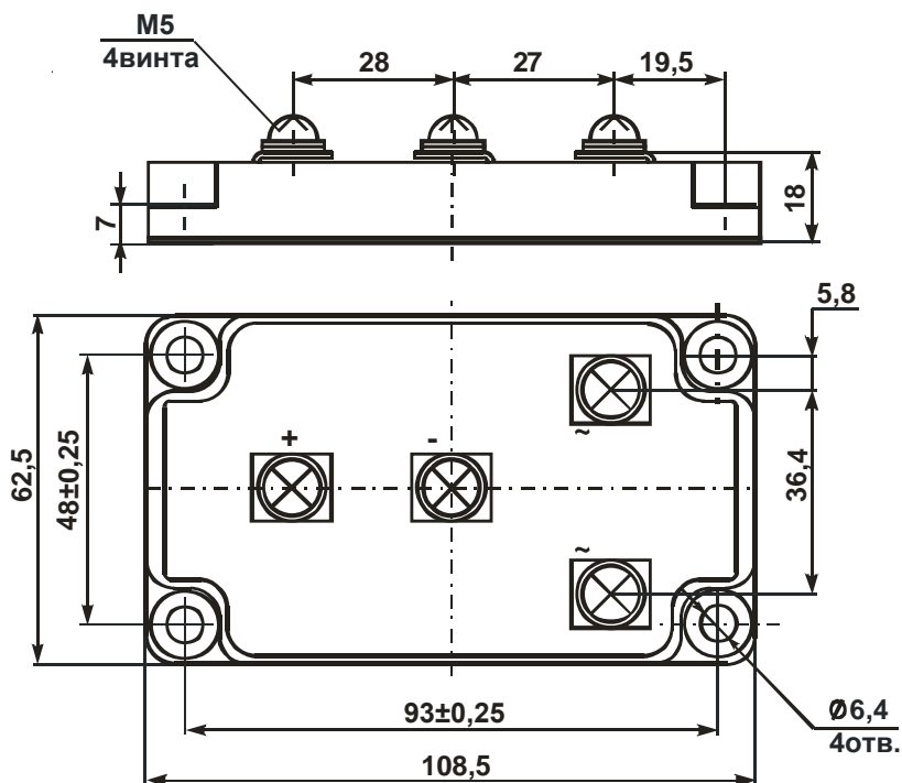
Рисунок 2 – Габаритные и присоединительные размеры
