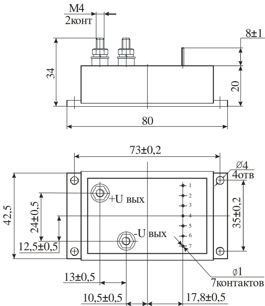
Рисунок 3 – Габаритный чертёж модуля
