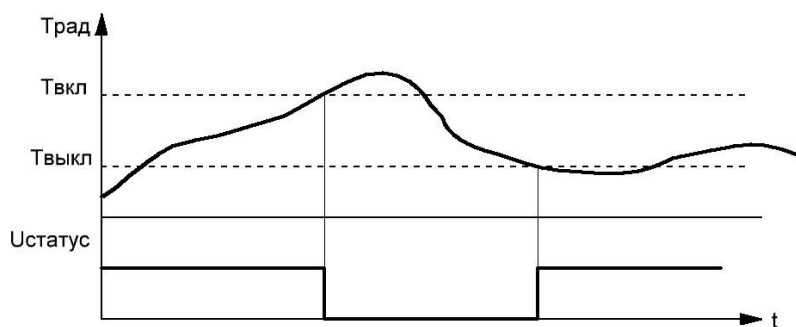
Рисунок 3 – Диаграмма функционирования температурной сигнализации
