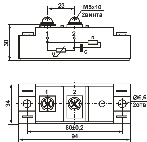
Рисунок 2 – модули MB2- 250, MB2- 460
