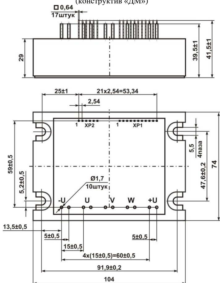
Рисунок 9.5 – Габаритные размеры М32-xx-xx-А-Д (конструктив «ДМ»)
