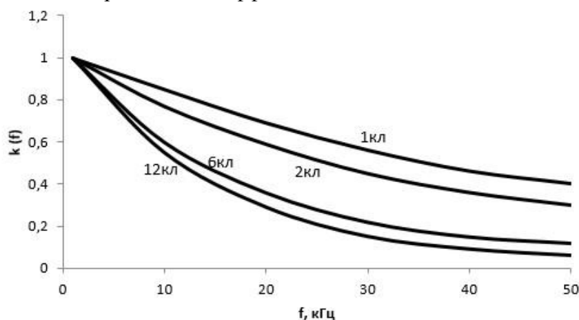
Рисунок 7.2 – Поправочный коэффициент k_F в зависимости от частоты
