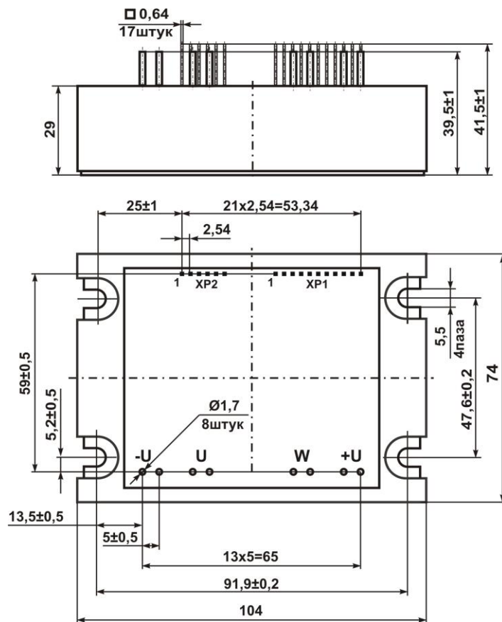
Рисунок 9.6 – Габаритные размеры М32-xx-xx-Б-Д (конструктив «ДМ»)
