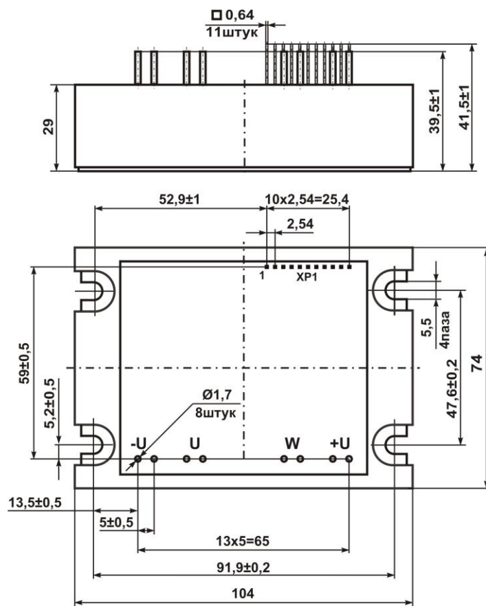
Рисунок 9.4 – Габаритные размеры М32-xx-xx-Б (конструктив «ДМ»)
