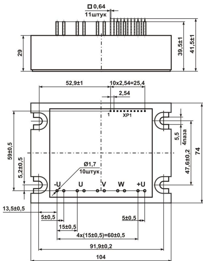
Рисунок 9.3 – Габаритные размеры М32-xx-xx-А (конструктив «ДМ»)
