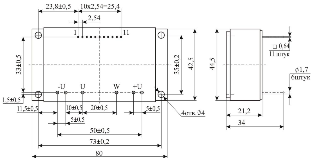
Рисунок 9.2 – Габаритные размеры М32-хх-хх-Б (конструктив «М»)
