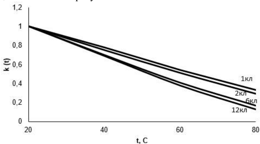
Рисунок 7.1 – Поправочный коэффициент k_T в зависимости от температуры
