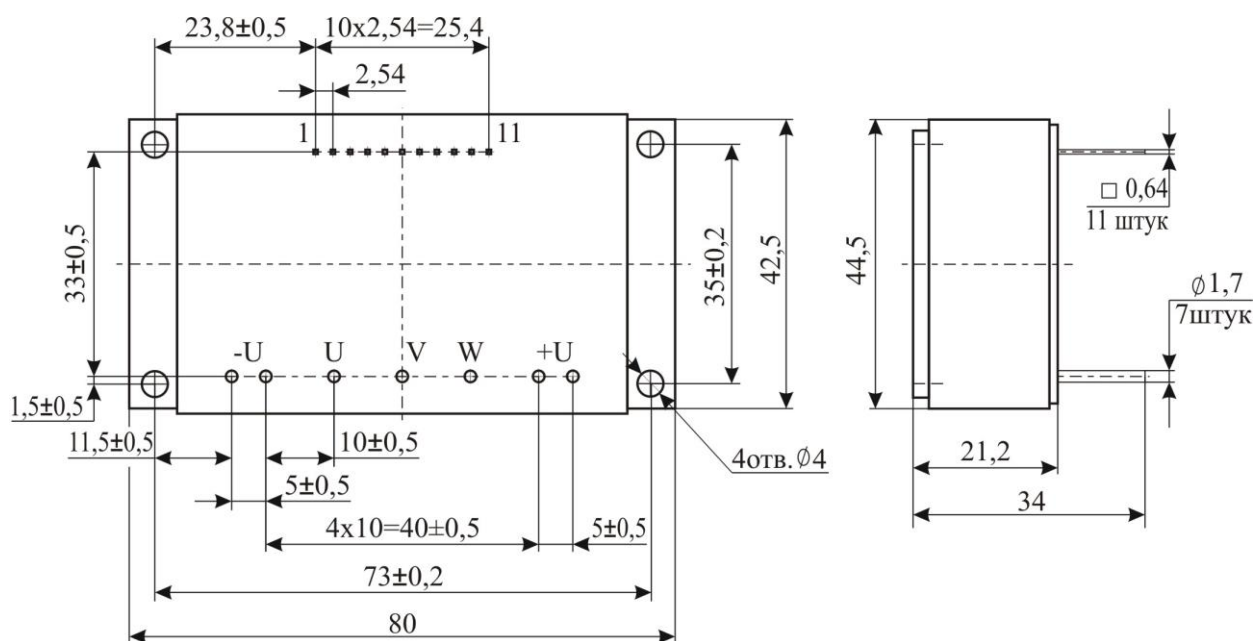
Рисунок 9.1 – Габаритные размеры М32-хх-хх-А (конструктив «М»)
