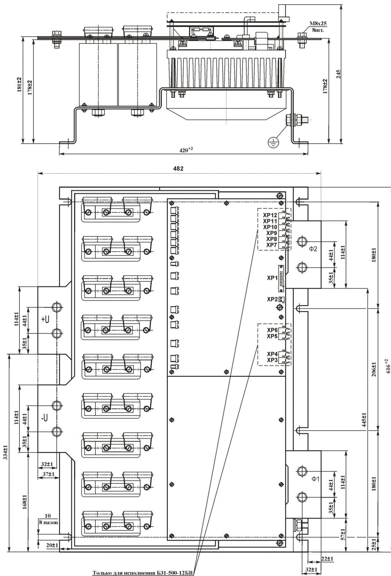
Рисунок 8.1 - Габаритные и присоединительные размеры блока
