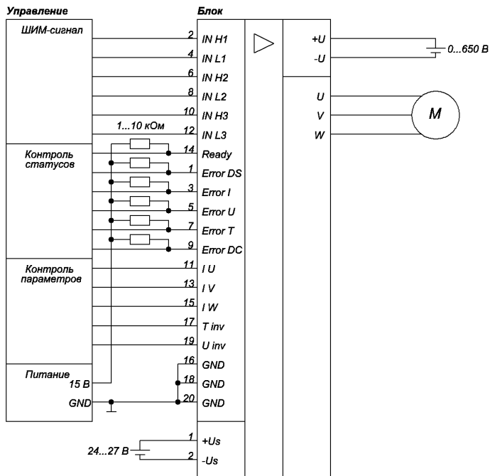
Рисунок 3.2 – Типовая схема включения Б31-500-12АП
