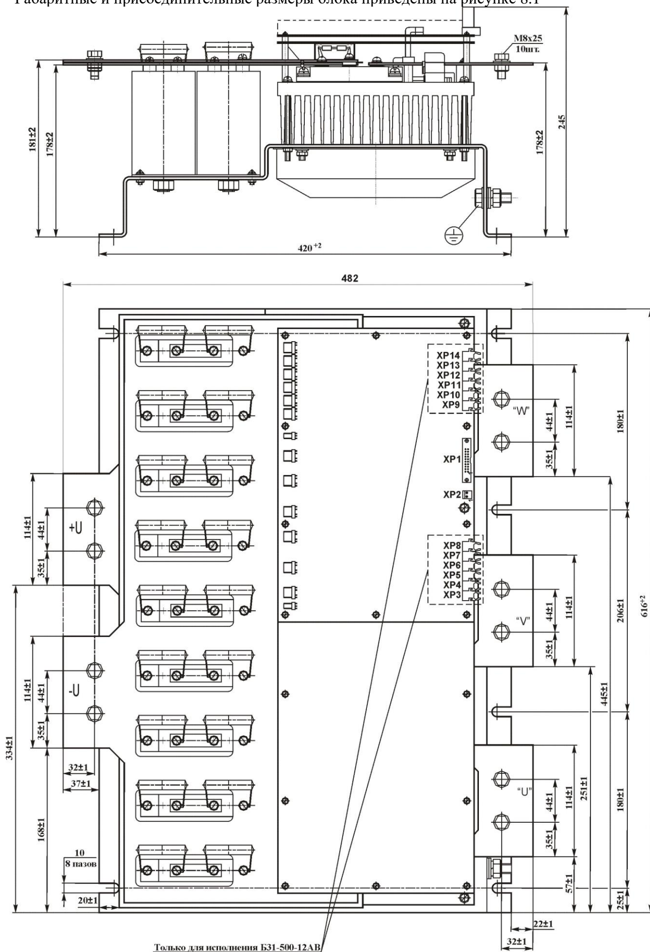
Рисунок 8.1 - Габаритные и присоединительные размеры блока
