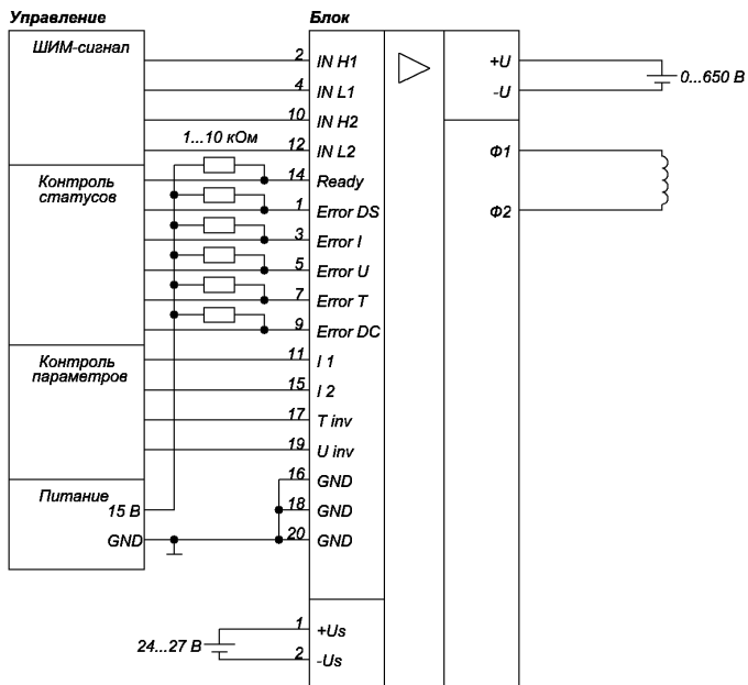
Рисунок 3.2 – Типовая схема включения Б31-300-12БП
