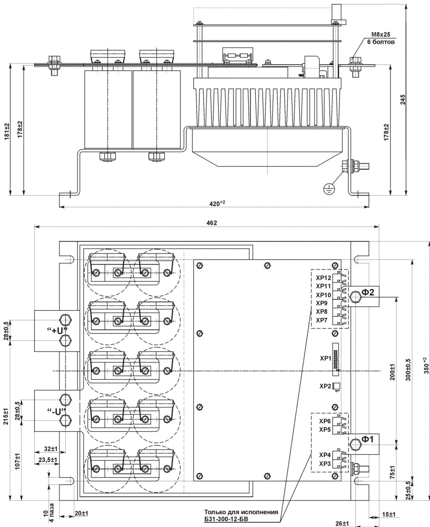
Рисунок 8.1 - Габаритные и присоединительные размеры блока
