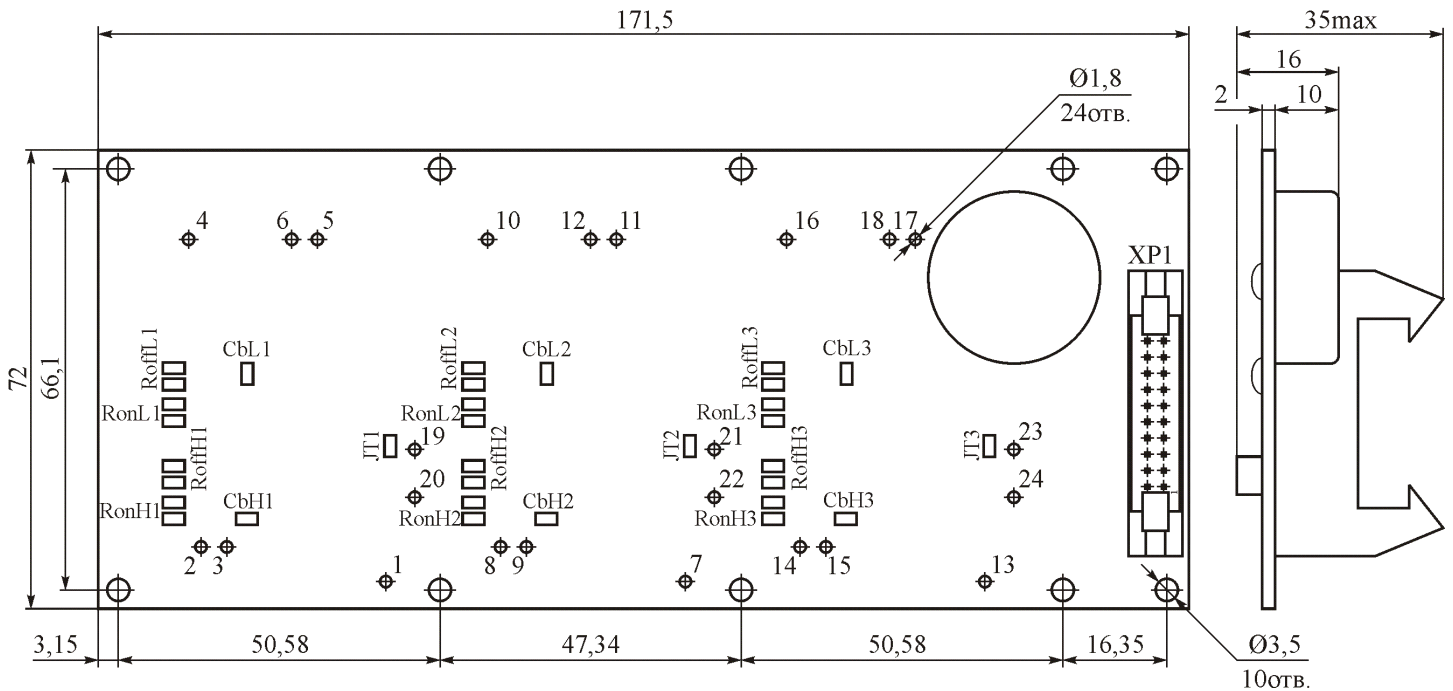
Рисунок 1 – Габаритный чертёж драйвера
