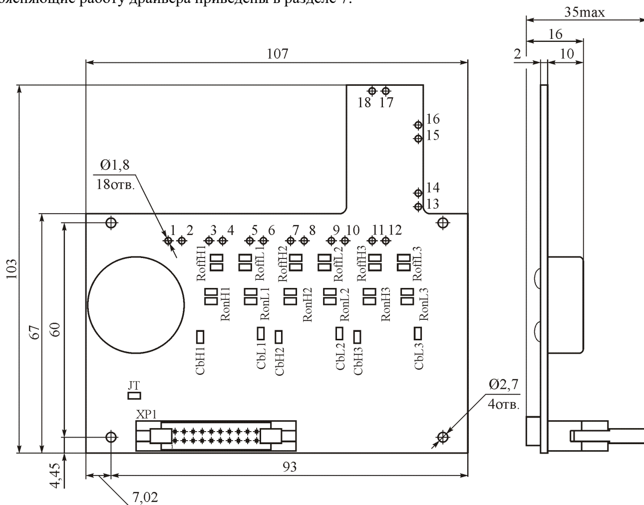
Рисунок 1 – Габаритный чертёж драйвера
