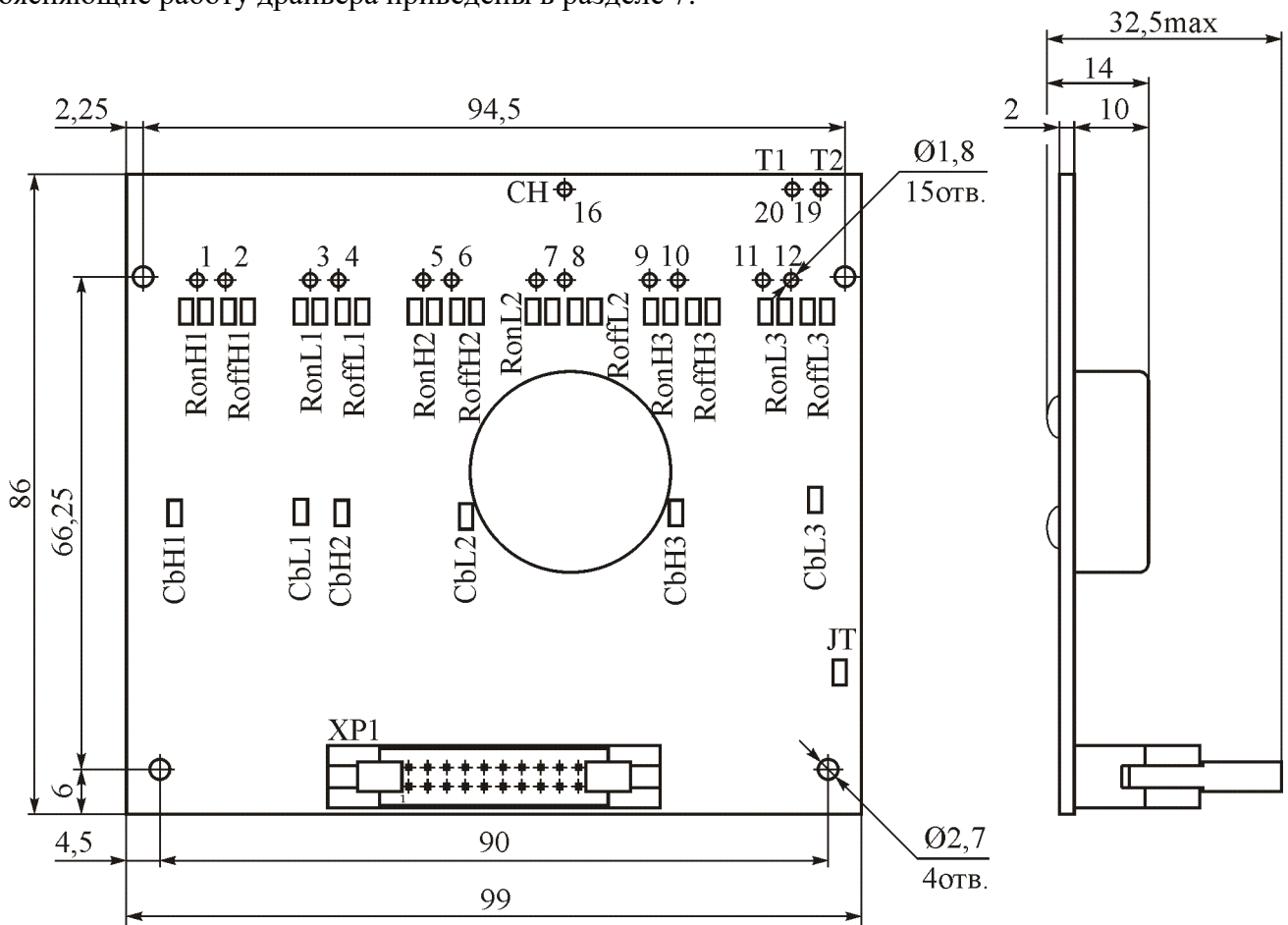
Рисунок 1 – Габаритный чертёж драйвера
