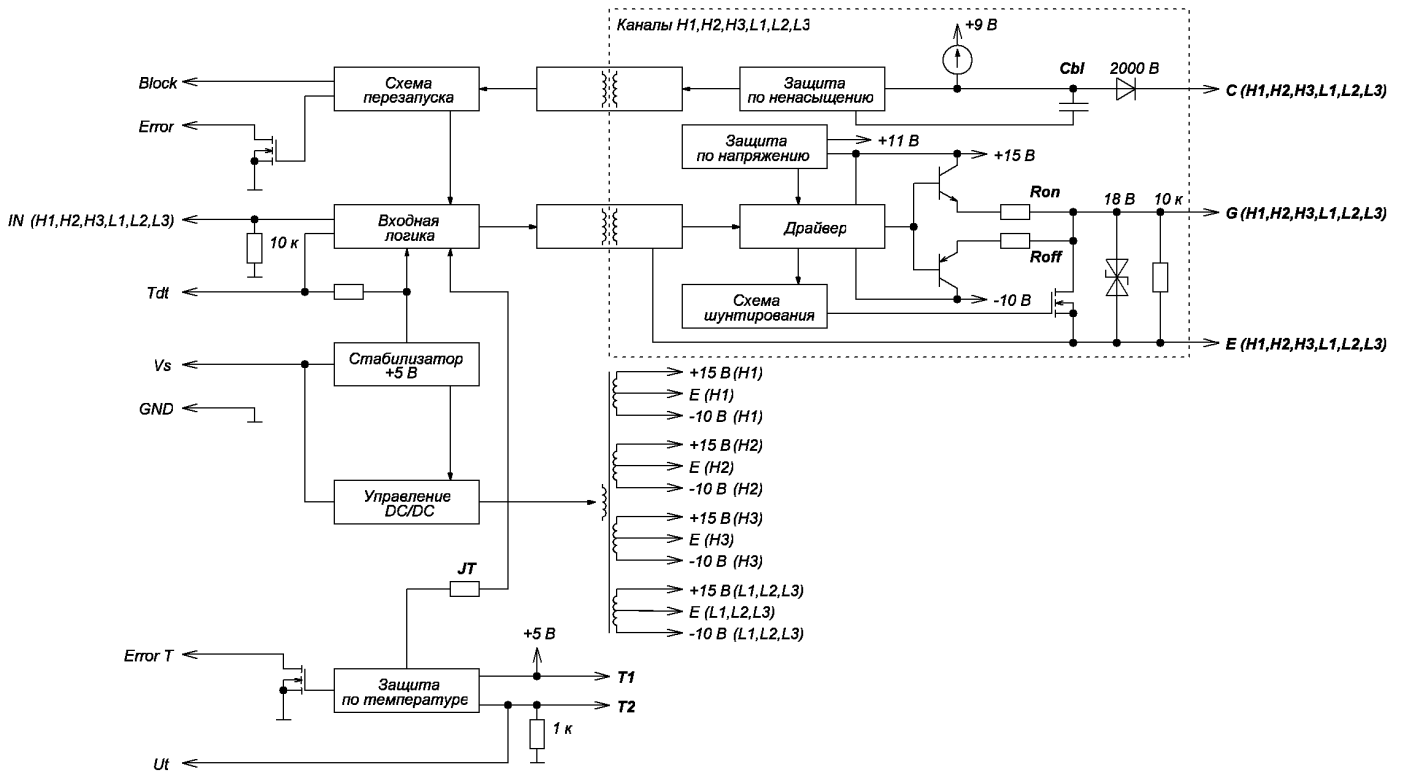
Рисунок 2– Структурная схема драйвера
