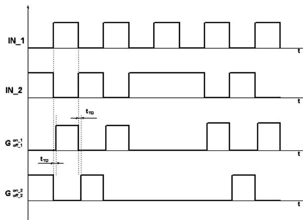
Рисунок 4 – Функциональная диаграмма работы драйвера
