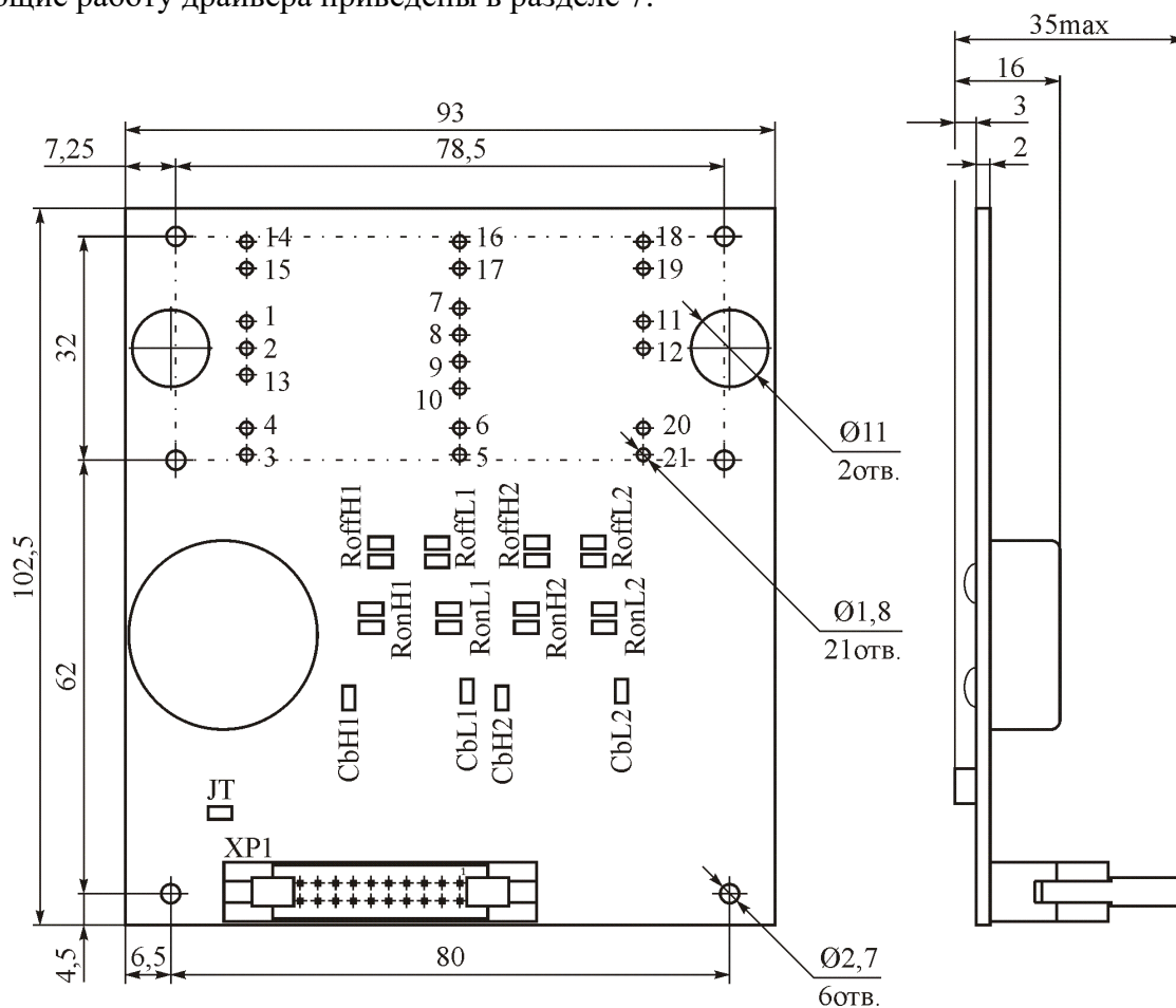
Рисунок 1 – Габаритный чертеж драйвера
