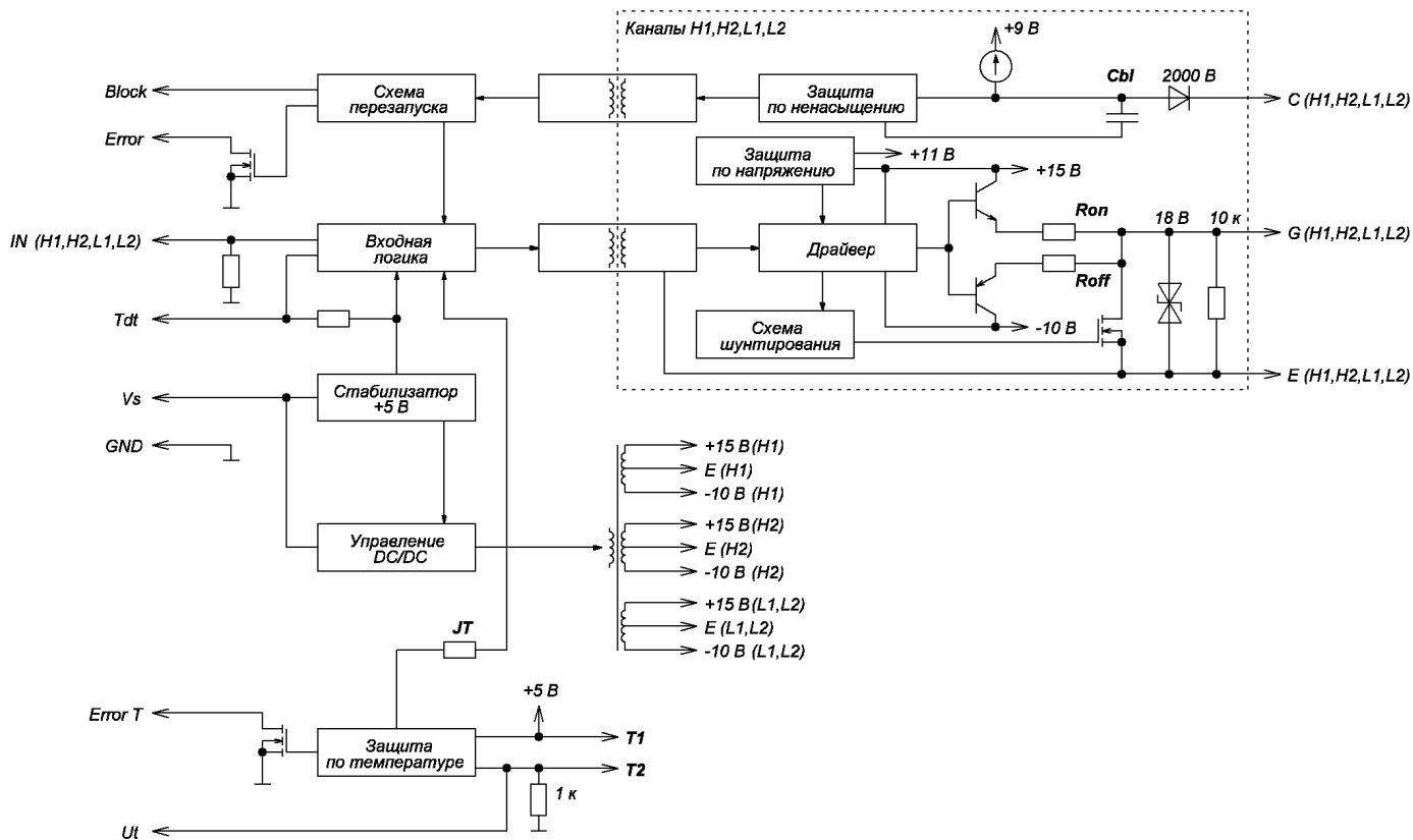
Рисунок 2– Структурная схема драйвера
