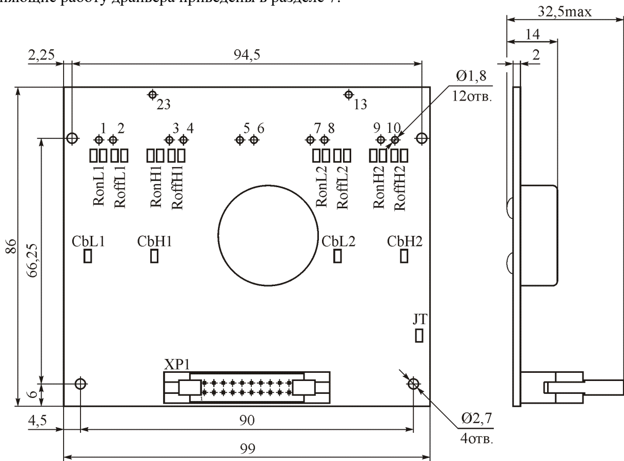
Рисунок 1 – Габаритный чертёж драйвера
