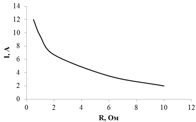
Рисунок 6 – График зависимости выходного импульсного тока от номинала затворных резисторов
