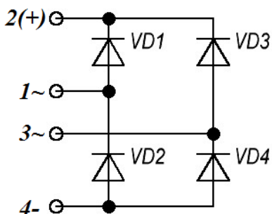
Рисунок 1 – Структурная схема модуля
